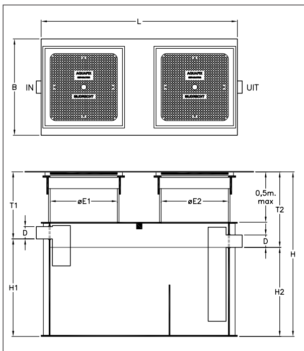
Afbeelding 2. Maattekening
