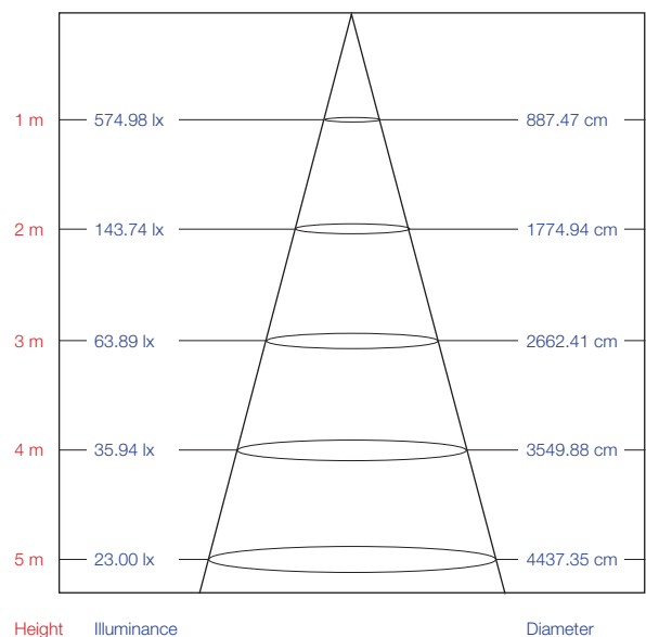
Lux-Distance Curve Voorbeeld type: Alta 20 W, 4000K
