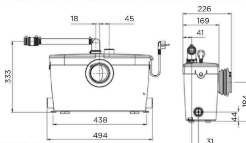
SANIACCESS® 3
