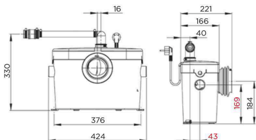
SANIACCESS® 1 - SANIACCESS® 2
