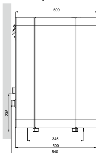
Zij-aanzicht
