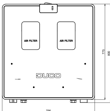
Vooraanzicht
