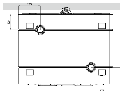
Onderaanzicht
