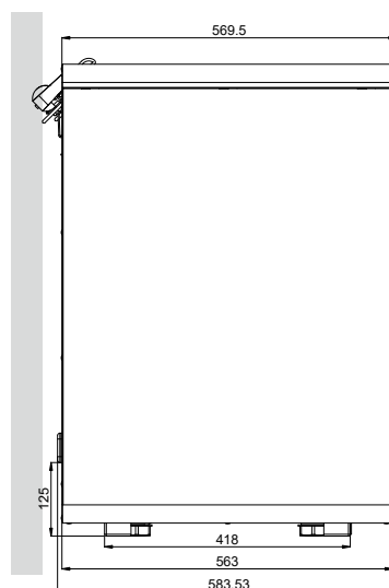
Zij-aanzicht
