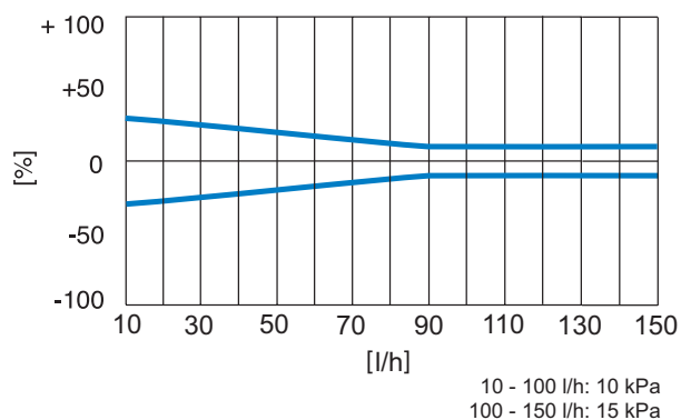
Minimale doorstromingstoleranties
