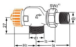
Axiaal met buitendraad G 3/4
