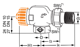
Axiaal
